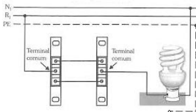
Diagrama funcional
